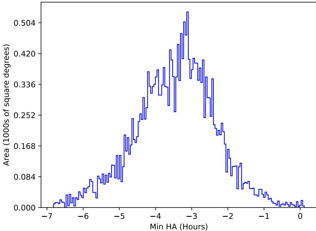
too_elab_r8_d2_ugrizy_v3.4_10yrs All sky y band: Min HA
