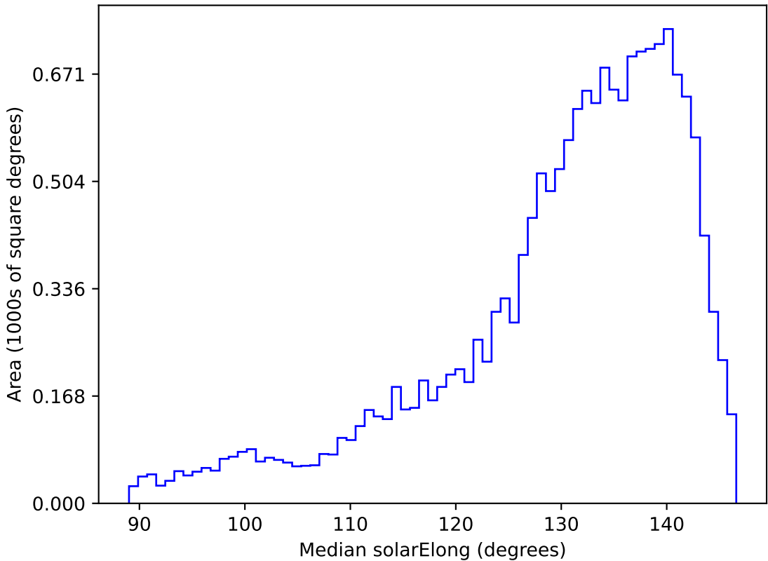
too_elab_r8_d2_ugrizy_v3.4_10yrs WFD y band: Median solarElong
