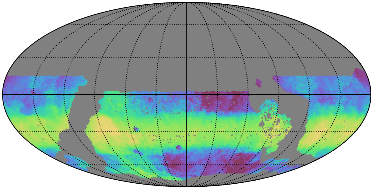
too_elab_r8_d2_ugrizy_v3.4_10yrs WFD y band: Median HA
