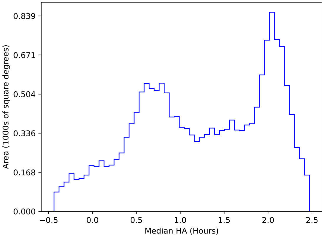
too_elab_r8_d2_ugrizy_v3.4_10yrs WFD y band: Median HA
