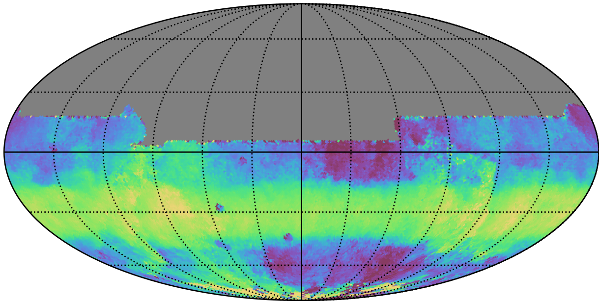
too_elab_r8_d2_ugrizy_v3.4_10yrs All sky y band: Median HA
