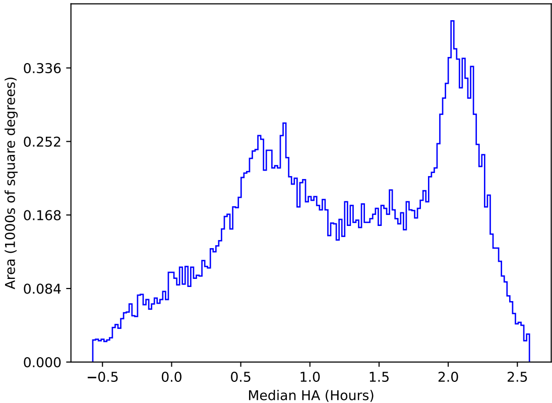
too_elab_r8_d2_ugrizy_v3.4_10yrs All sky y band: Median HA
