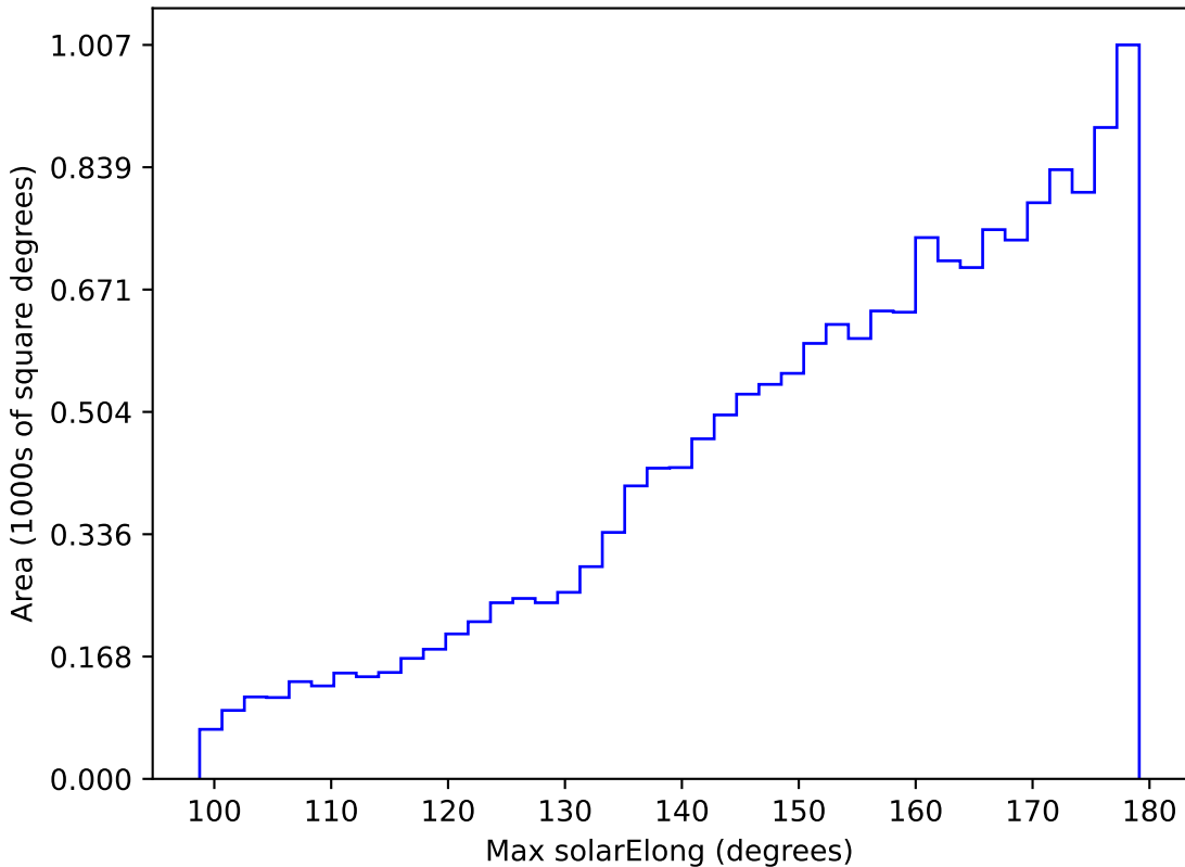
too_elab_r8_d2_ugrizy_v3.4_10yrs WFD y band: Max solarElong
