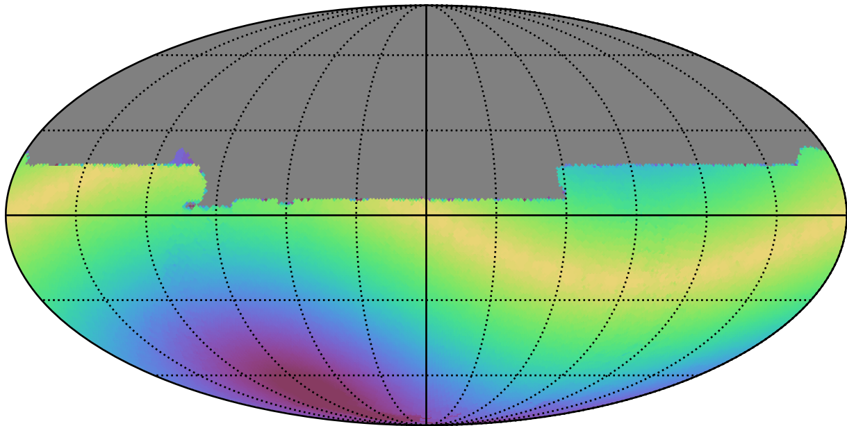
too_elab_r8_d2_ugrizy_v3.4_10yrs All sky y band: Max solarElong
