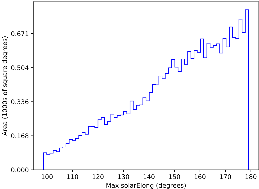
too_elab_r8_d2_ugrizy_v3.4_10yrs All sky y band: Max solarElong
