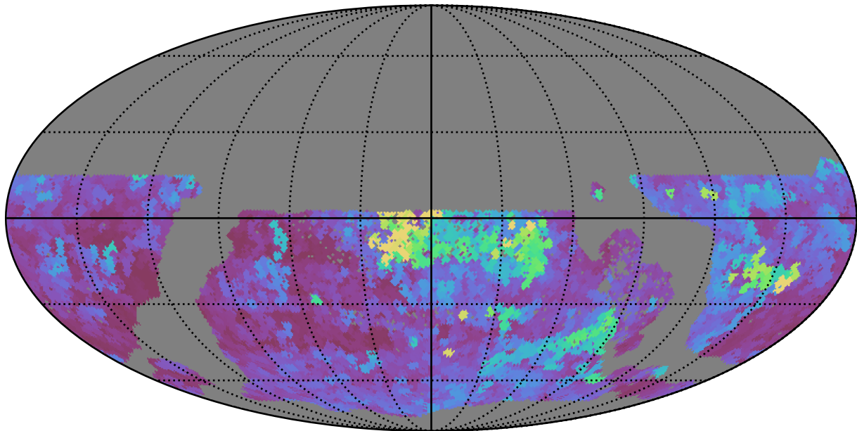
too_elab_r8_d2_ugrizy_v3.4_10yrs WFD y band: Max seeingEff
