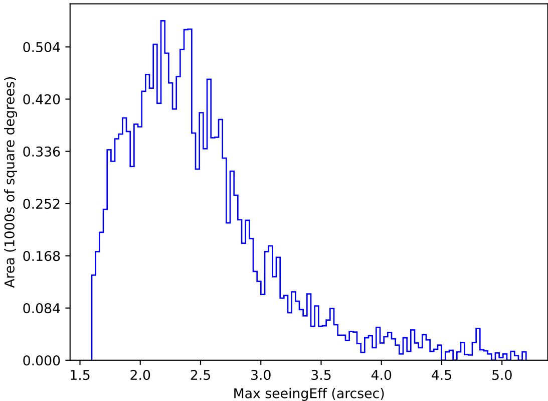
too_elab_r8_d2_ugrizy_v3.4_10yrs WFD y band: Max seeingEff
