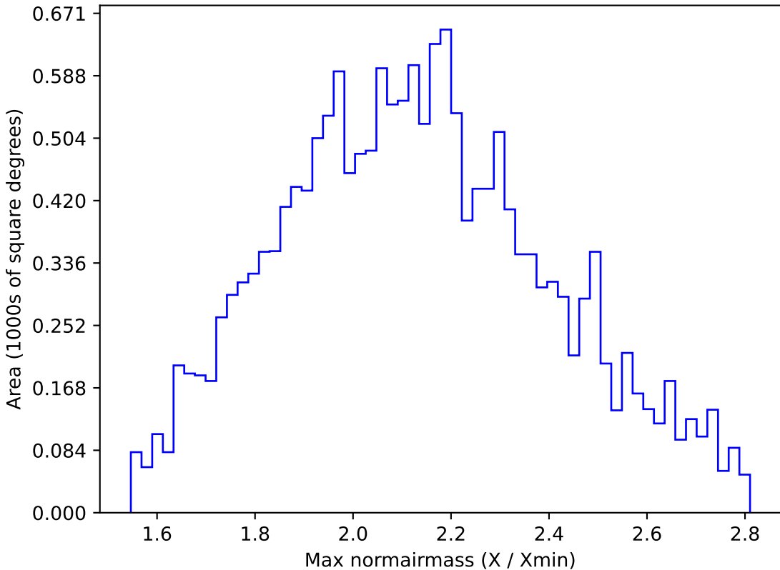
too_elab_r8_d2_ugrizy_v3.4_10yrs WFD y band: Max normairmass
