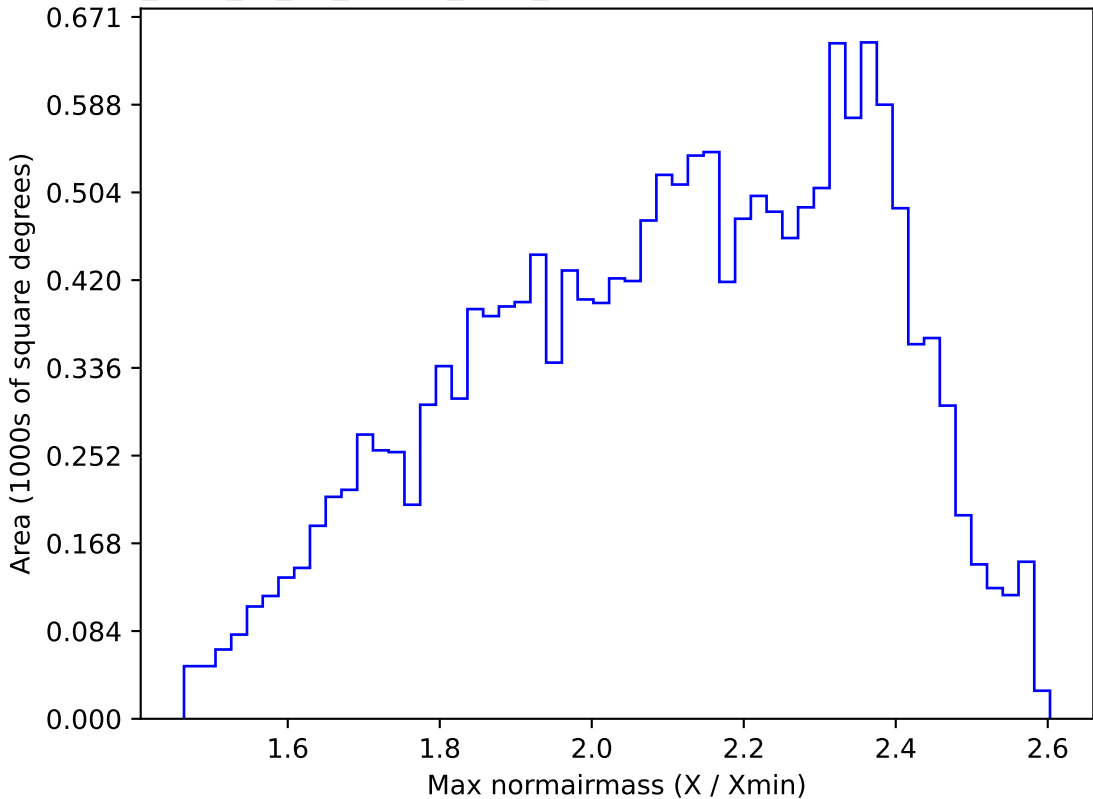
too_elab_r8_d2_ugrizy_v3.4_10yrs WFD r band: Max normairmass
