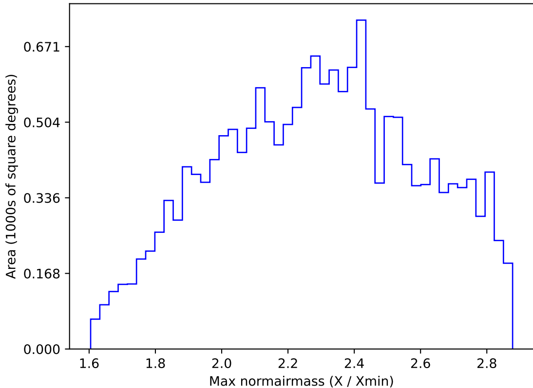
too_elab_r8_d2_ugrizy_v3.4_10yrs WFD i band: Max normairmass
