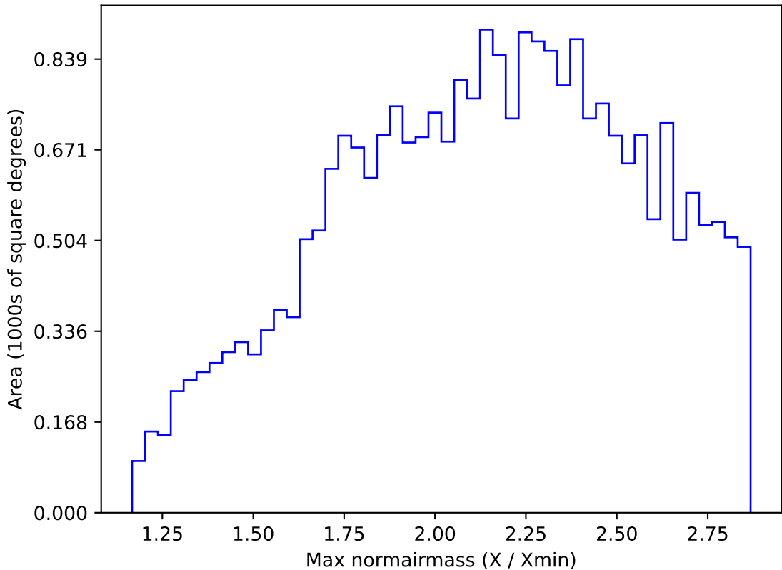
too_elab_r8_d2_ugrizy_v3.4_10yrs All sky z band: Max normairmass
