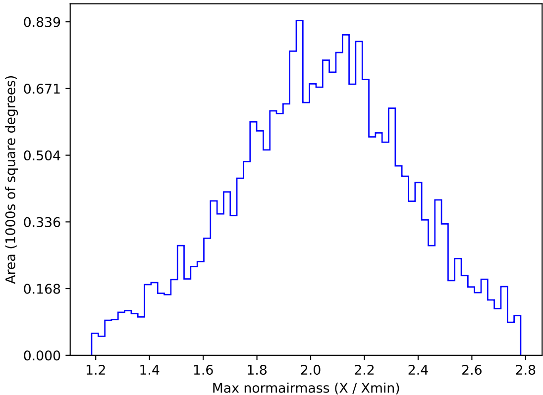
too_elab_r8_d2_ugrizy_v3.4_10yrs All sky y band: Max normairmass
