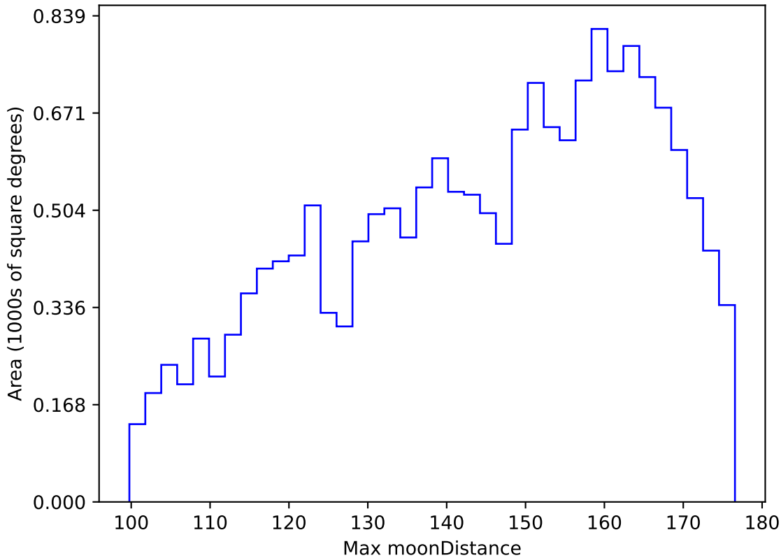
too_elab_r8_d2_ugrizy_v3.4_10yrs WFD y band: Max moonDistance
