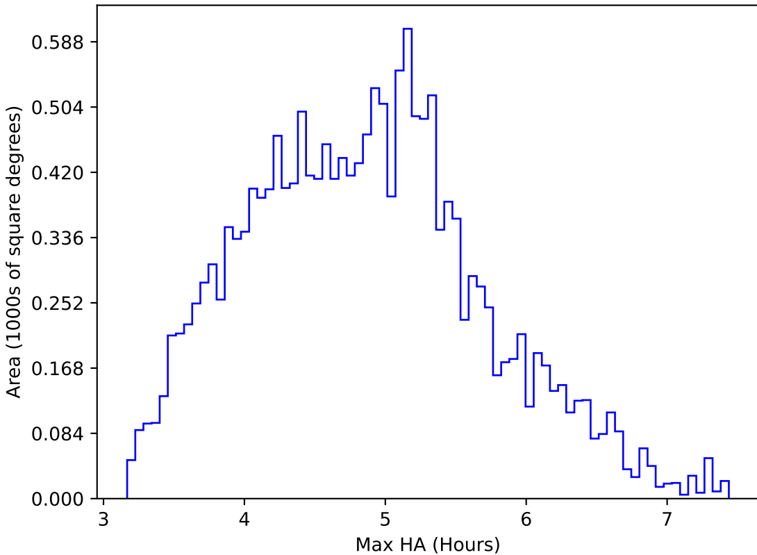
too_elab_r8_d2_ugrizy_v3.4_10yrs WFD z band: Max HA
