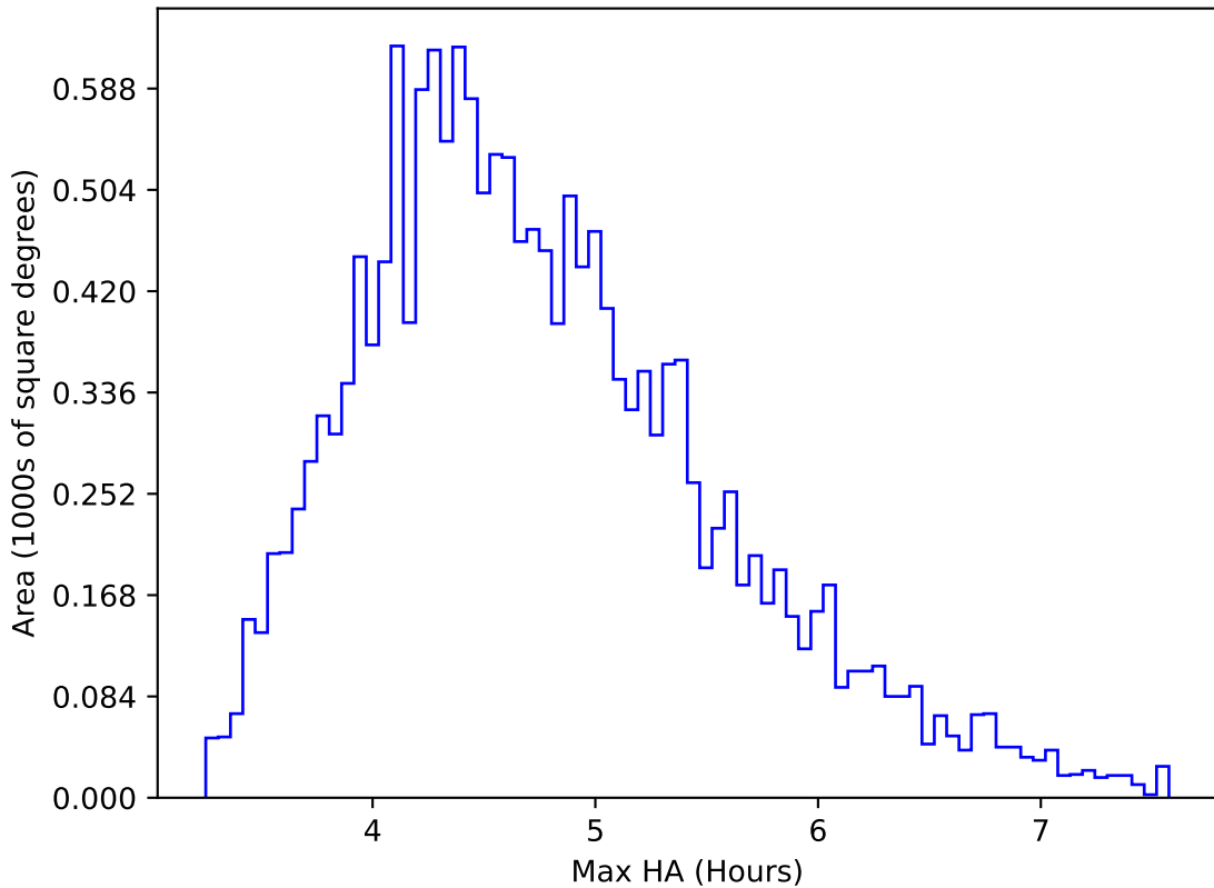
too_elab_r8_d2_ugrizy_v3.4_10yrs WFD y band: Max HA
