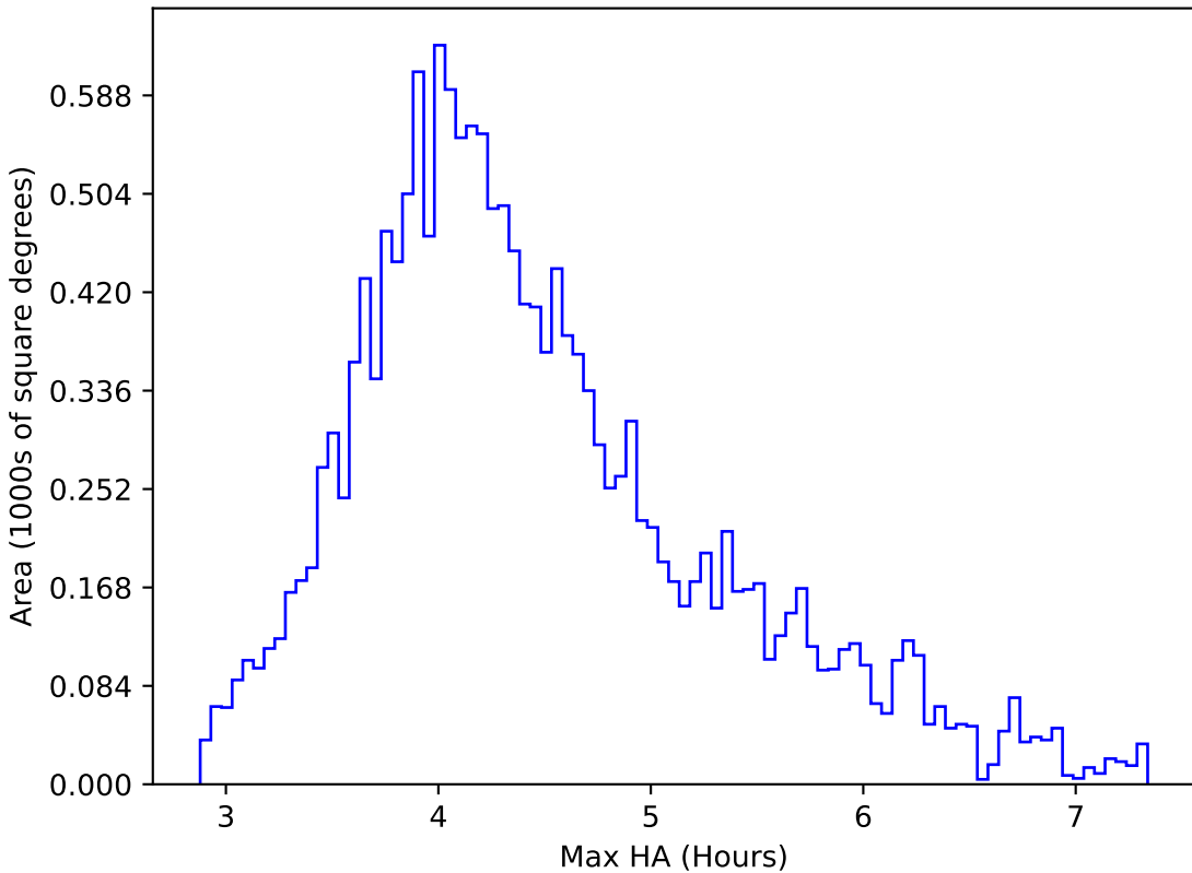
too_elab_r8_d2_ugrizy_v3.4_10yrs WFD r band: Max HA
