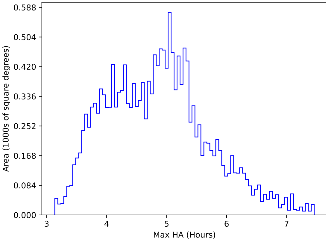
too_elab_r8_d2_ugrizy_v3.4_10yrs WFD i band: Max HA
