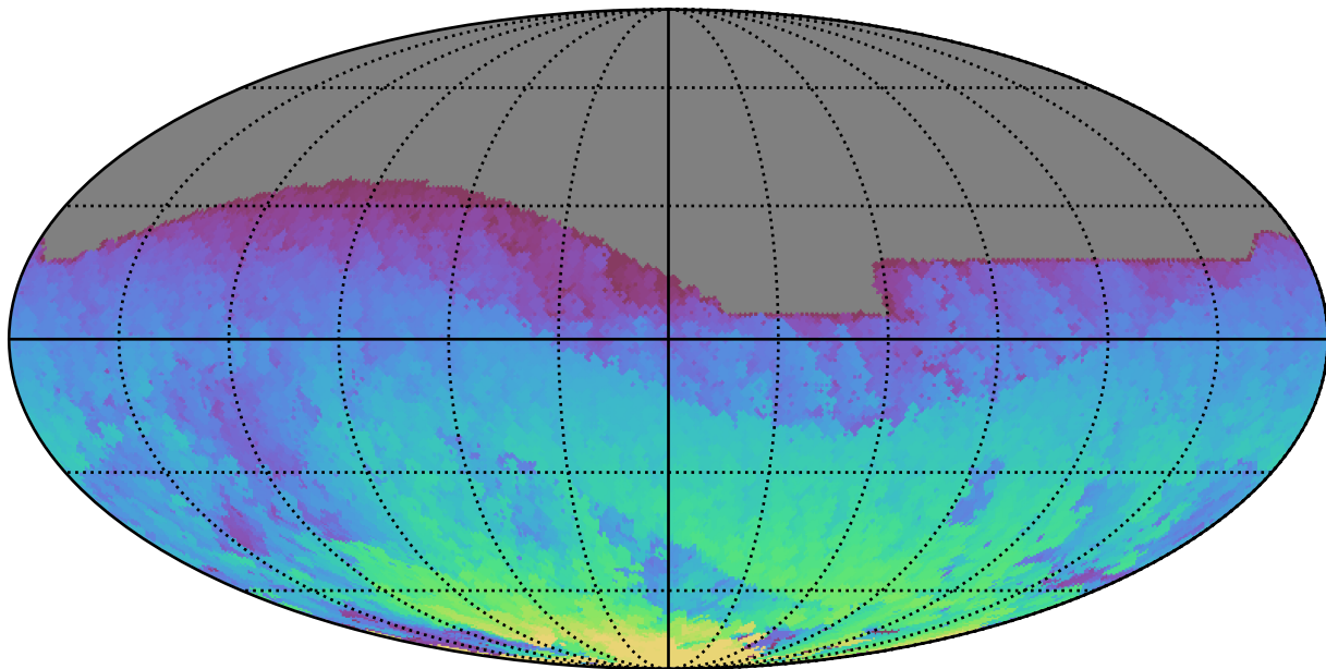
too_elab_r8_d2_ugrizy_v3.4_10yrs All sky z band: Max HA
