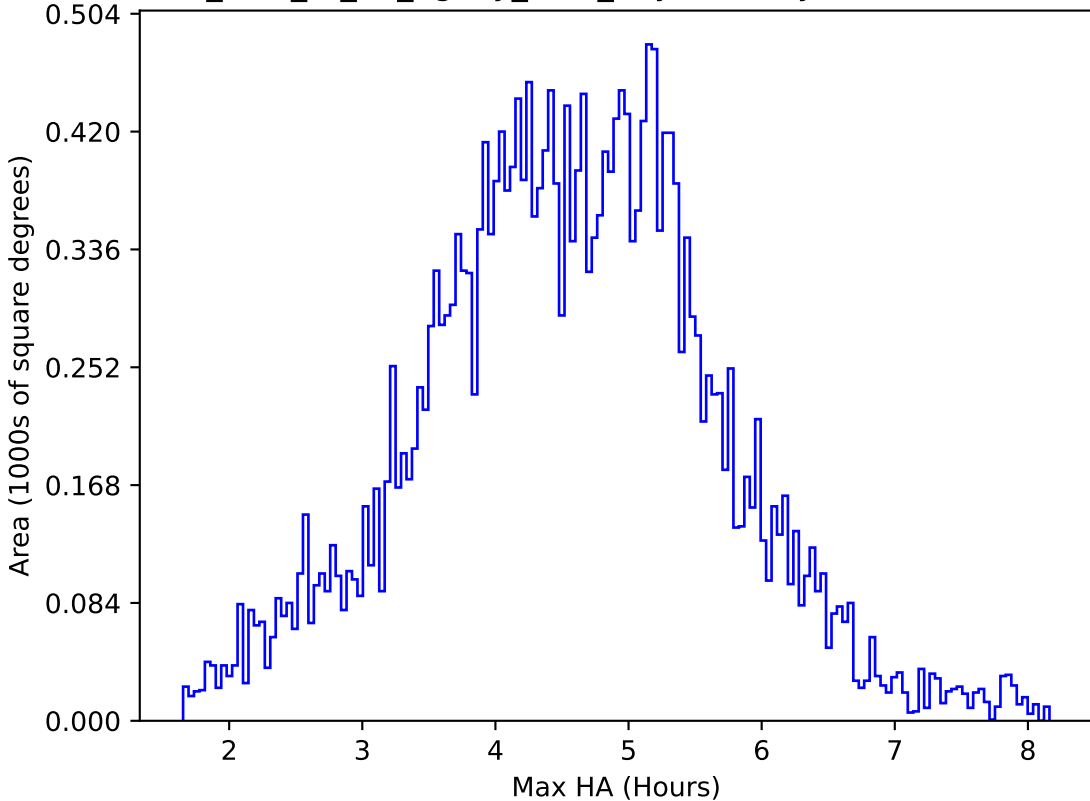
too_elab_r8_d2_ugrizy_v3.4_10yrs All sky z band: Max HA
