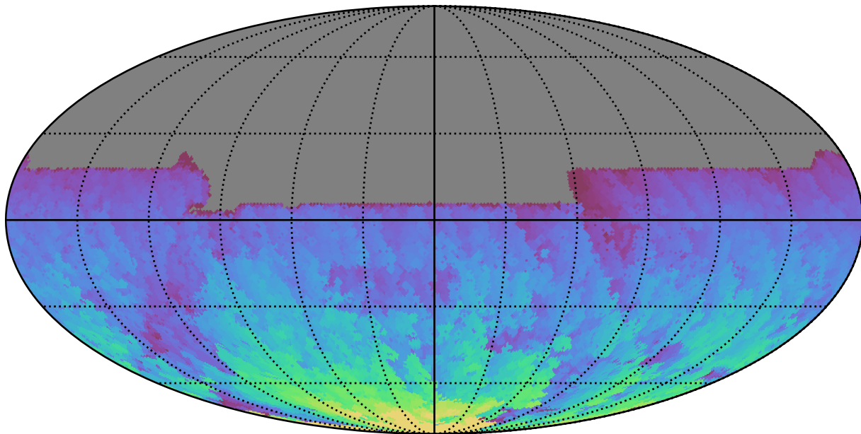
too_elab_r8_d2_ugrizy_v3.4_10yrs All sky y band: Max HA
