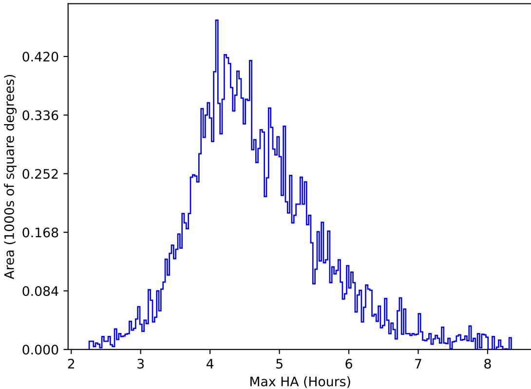
too_elab_r8_d2_ugrizy_v3.4_10yrs All sky y band: Max HA
