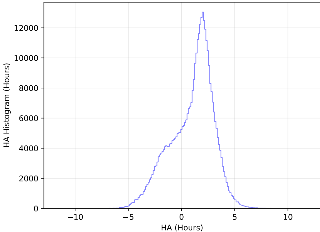
too_elab_r8_d2_ugrizy_v3.4_10yrs WFD y band: HA Histogram
