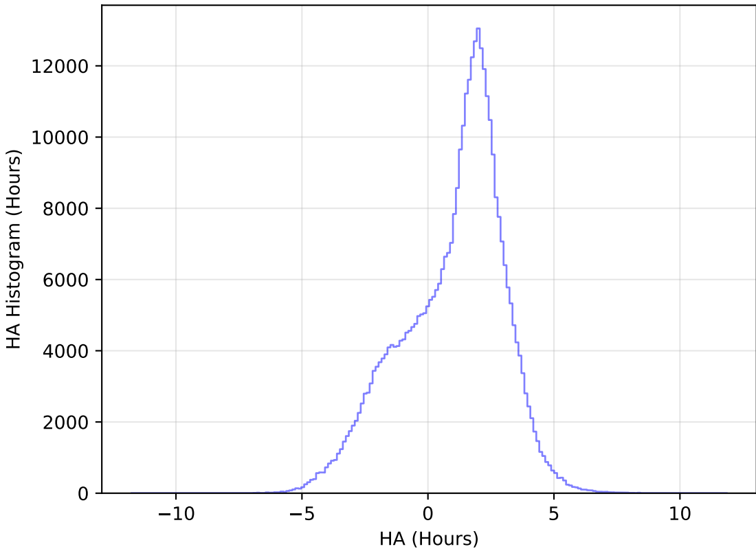
too_elab_r8_d2_ugrizy_v3.4_10yrs All sky y band: HA Histogram
