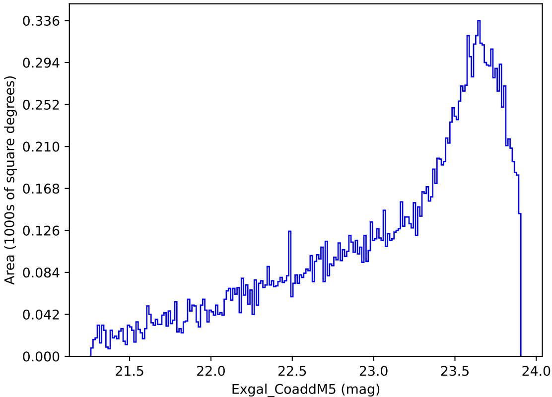
too_elab_r8_d2_ugrizy_v3.4_10yrs Yr 3-4 y band: Exgal_CoaddM5
