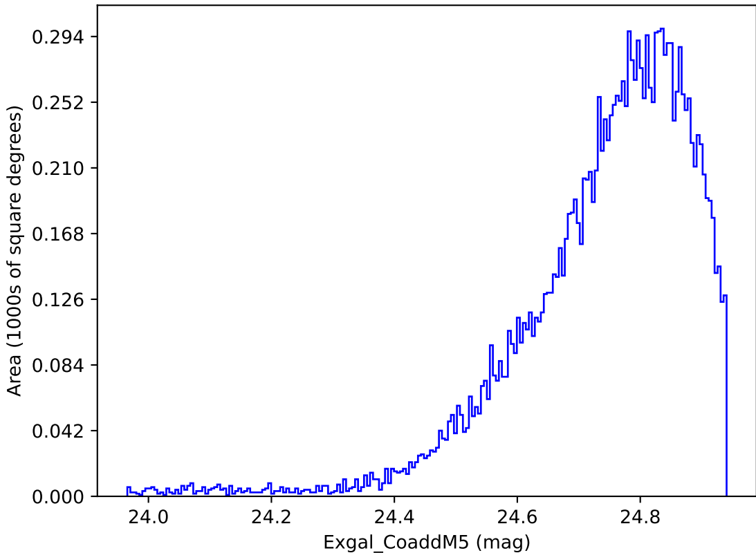
too_elab_r8_d2_ugrizy_v3.4_10yrs WFD y band: Exgal_CoaddM5
