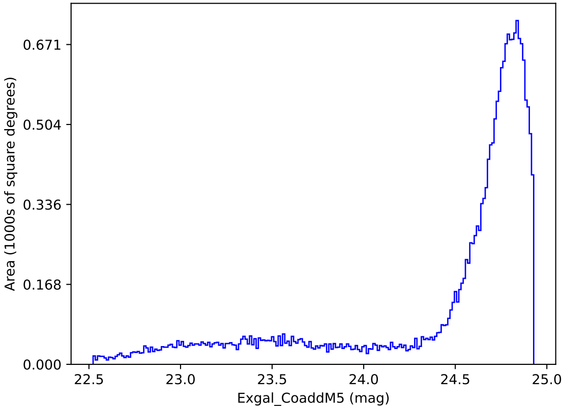
too_elab_r8_d2_ugrizy_v3.4_10yrs All sky y band: Exgal_CoaddM5
