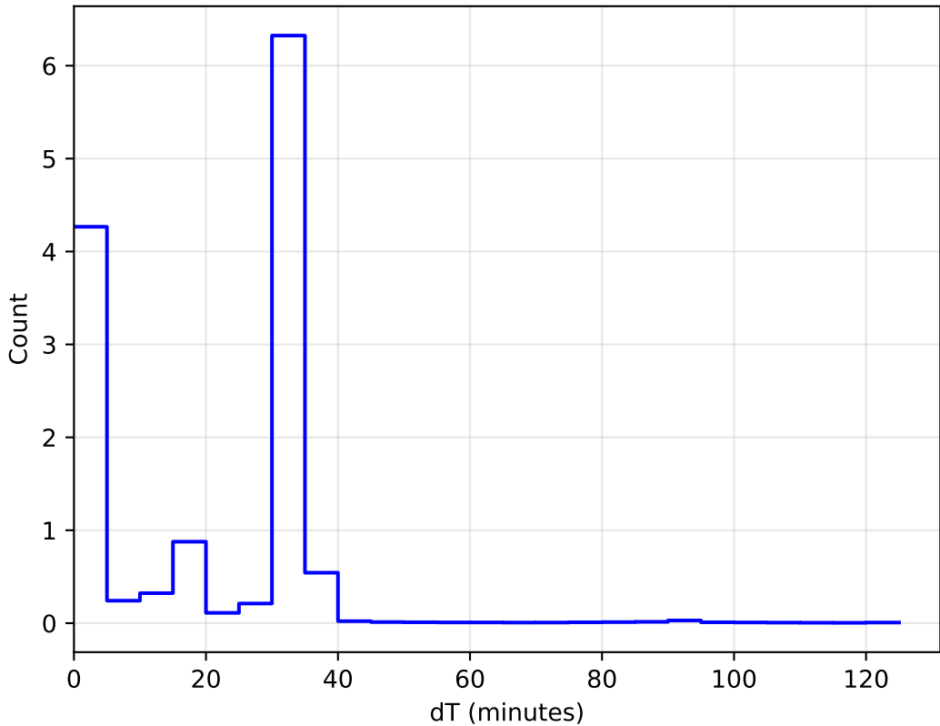
too_elab_r8_d2_ugrizy_v3.4_10yrs All sky: DeltaT Histogram 1e6
