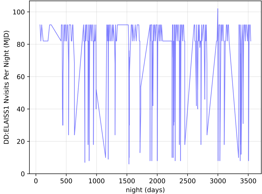
too_elab_r8_d2_ugrizy_v3.4_10yrs all bands: DD:ELAISS1 Nvisits Per Night
