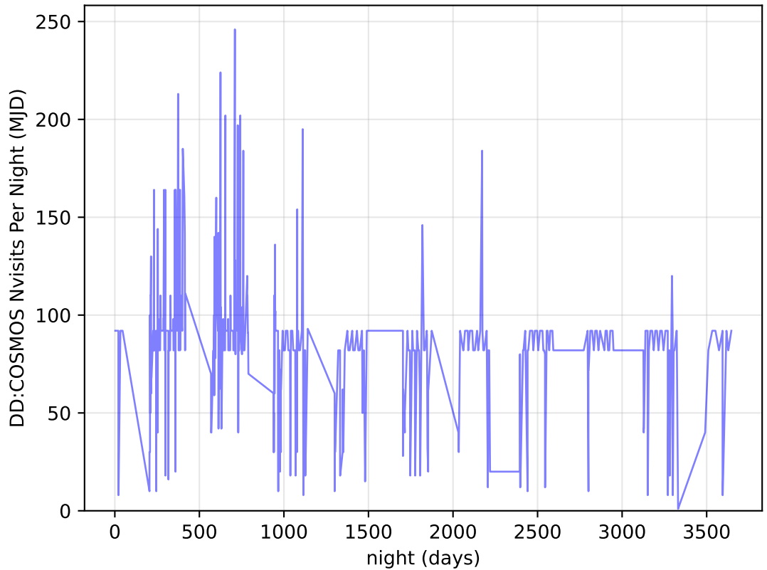
too_elab_r8_d2_ugrizy_v3.4_10yrs all bands: DD:COSMOS Nvisits Per Night
