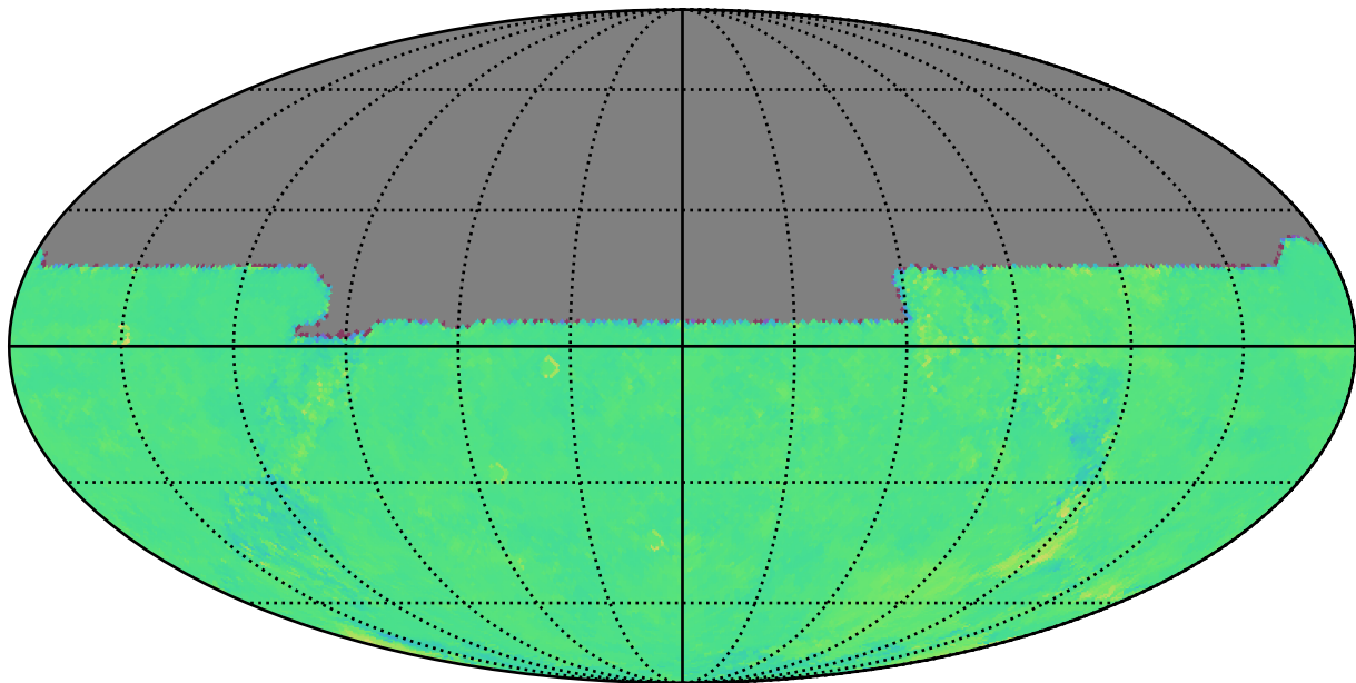
too_elab_r8_d2_gz_v3.4_10yrs u: Kuiper rotTelPos
