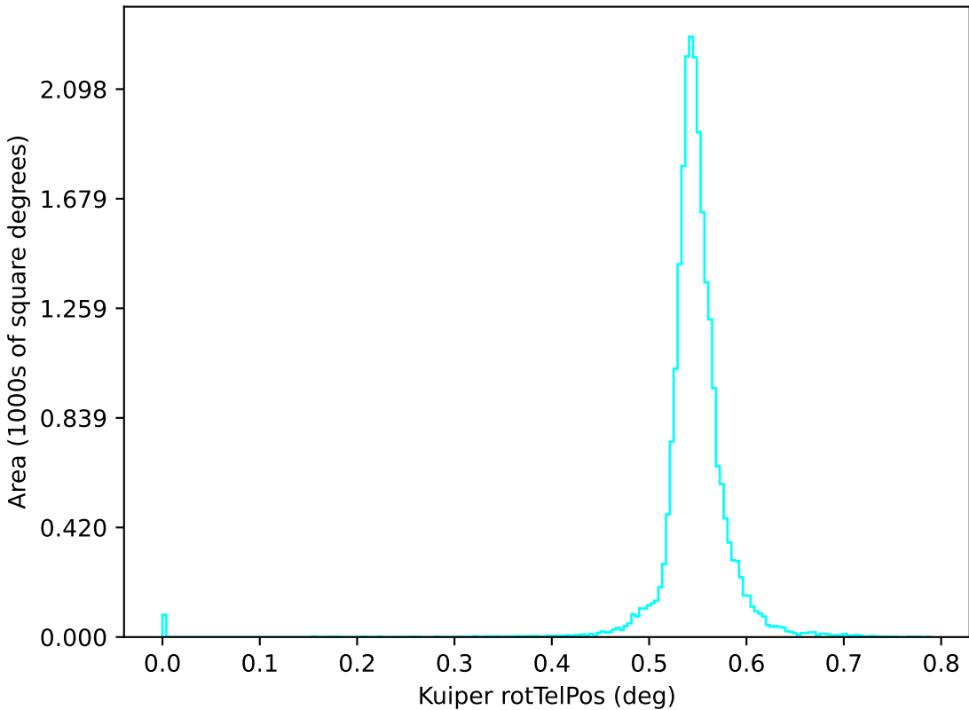
too_elab_r8_d2_gz_v3.4_10yrs u: Kuiper rotTelPos
