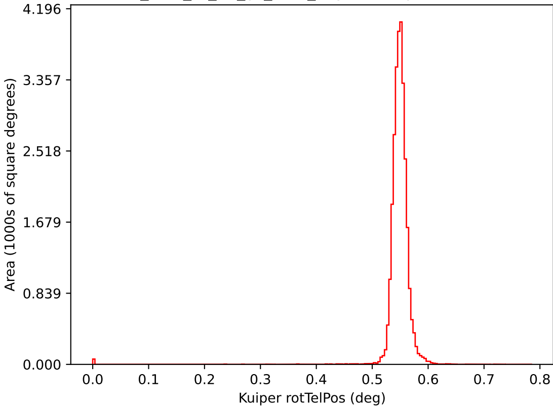
too_elab_r8_d2_gz_v3.4_10yrs i: Kuiper rotTelPos
