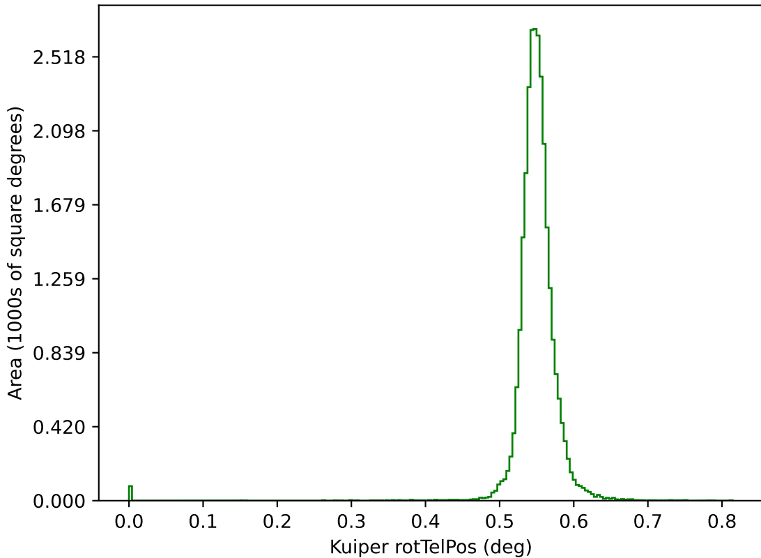
too_elab_r8_d2_gz_v3.4_10yrs g: Kuiper rotTelPos
