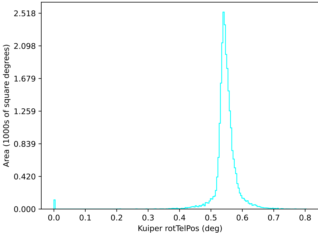
too_elab_r8_d2_griz_v3.4_10yrs u: Kuiper rotTelPos
