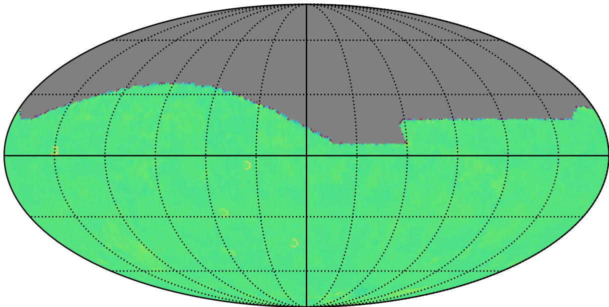
too_elab_r8_d2_griz_v3.4_10yrs i: Kuiper rotTelPos
