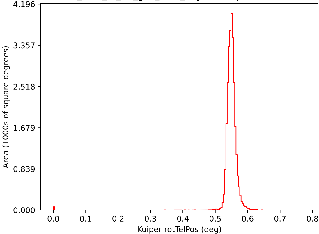
too_elab_r8_d2_griz_v3.4_10yrs i: Kuiper rotTelPos
