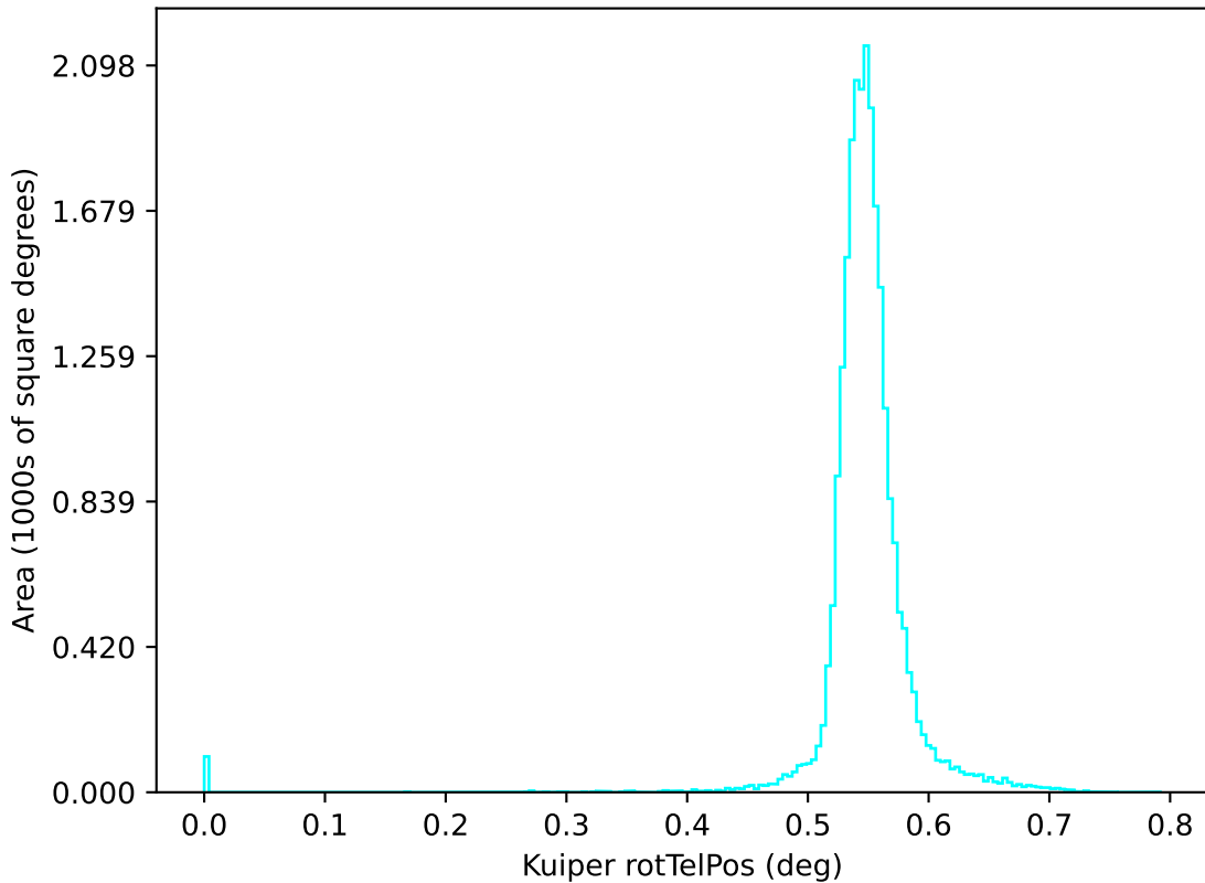
too_elab_r8_d2_giz_v3.4_10yrs u: Kuiper rotTelPos
