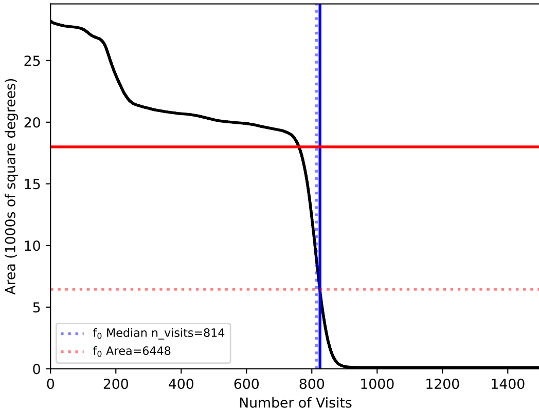
too_elab_r64_d3_ugrizy_v3.4_10yrs : f0
