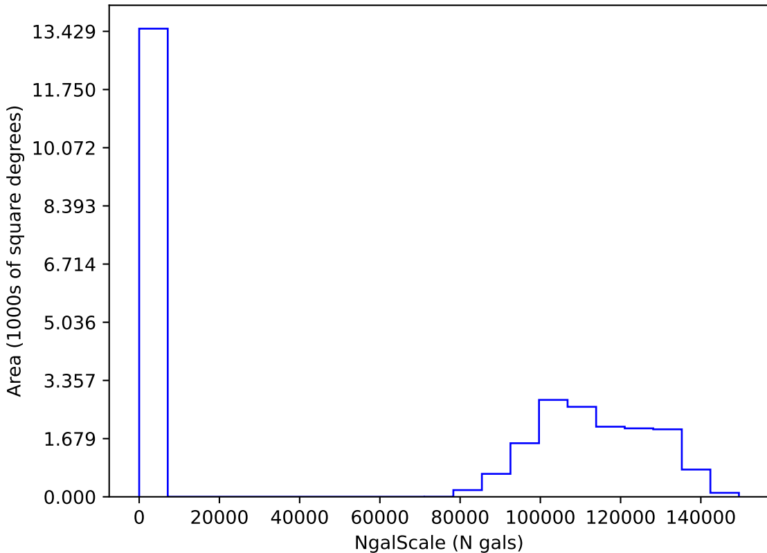
too_elab_r64_d3_ugrizy_v3.4_10yrs i: NgalScale
