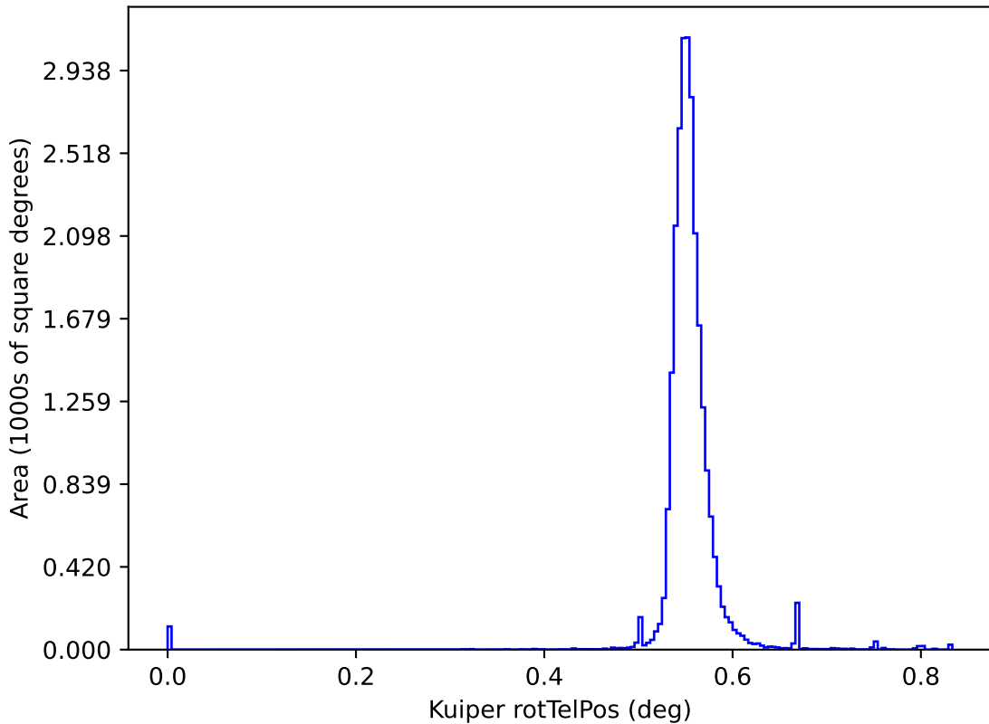
too_elab_r64_d3_ugrizy_v3.4_10yrs y: Kuiper rotTelPos
