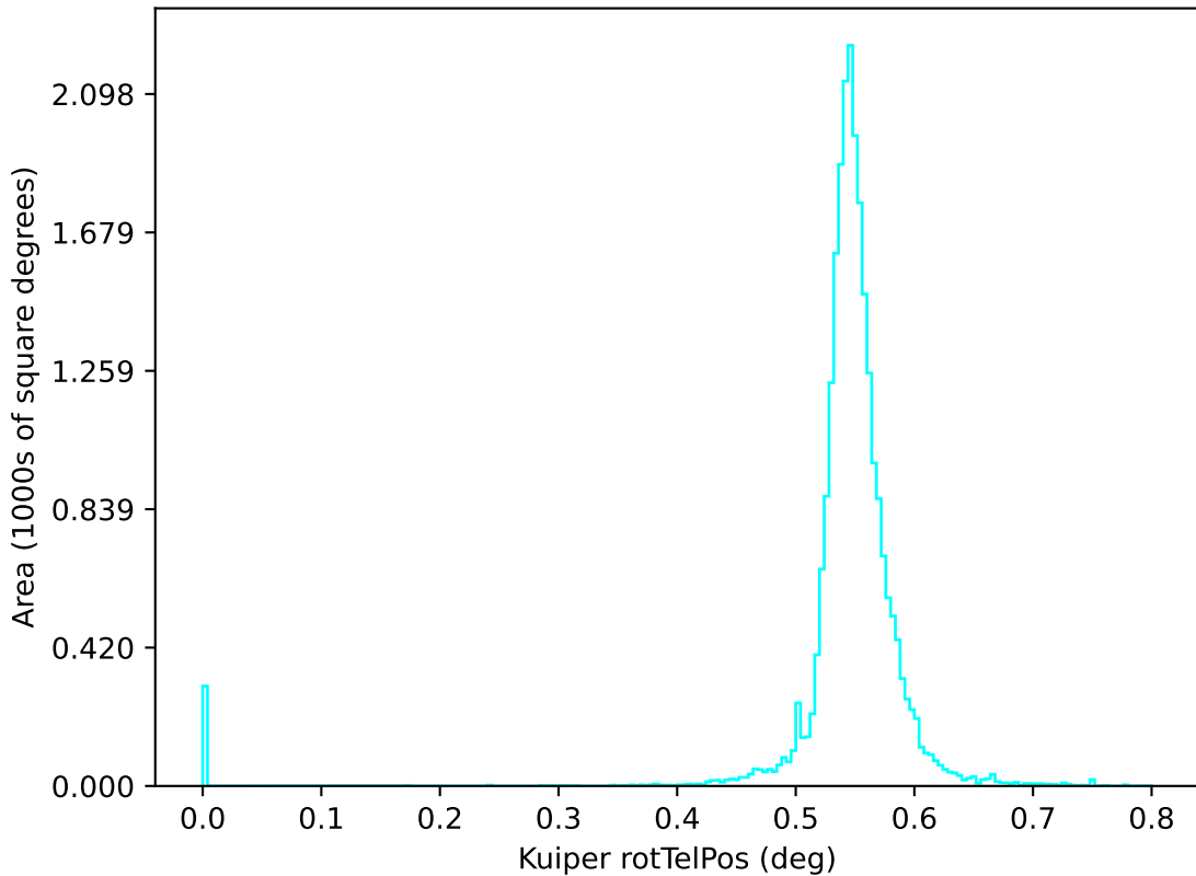
too_elab_r64_d3_ugrizy_v3.4_10yrs u: Kuiper rotTelPos
