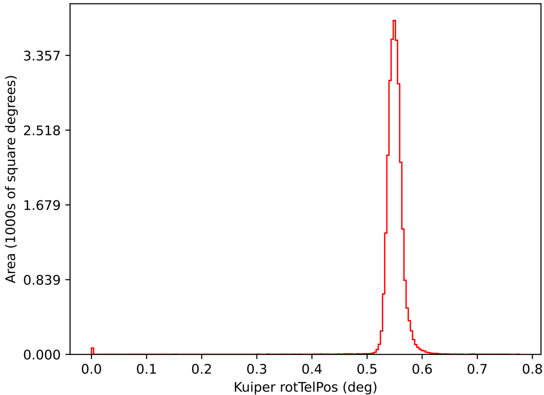
too_elab_r64_d3_ugrizy_v3.4_10yrs i: Kuiper rotTelPos
