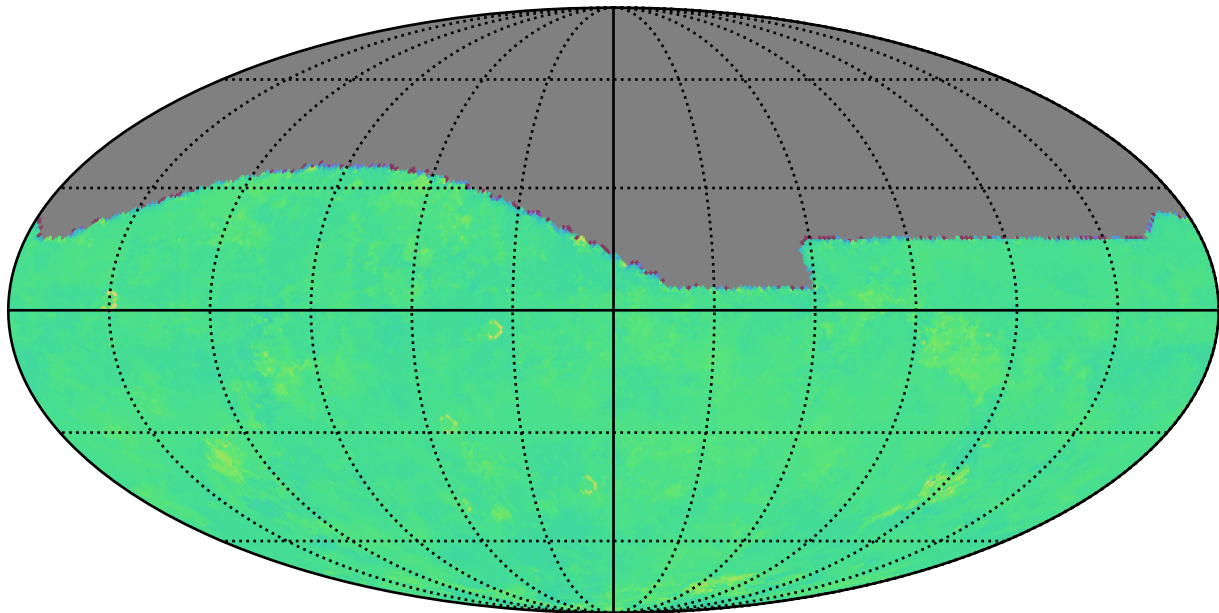
too_elab_r64_d3_ugrizy_v3.4_10yrs g: Kuiper rotTelPos
