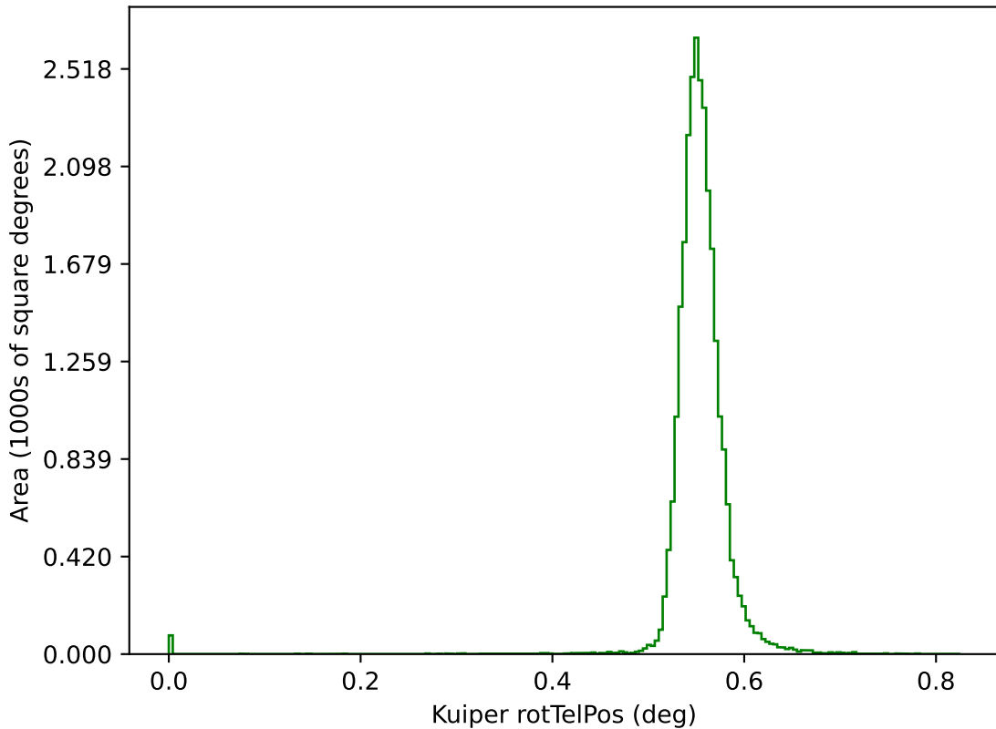
too_elab_r64_d3_ugrizy_v3.4_10yrs g: Kuiper rotTelPos
