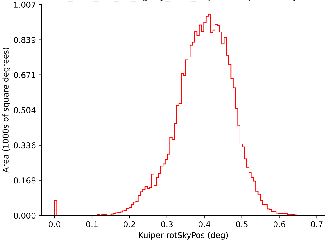
too_elab_r64_d3_ugrizy_v3.4_10yrs i: Kuiper rotSkyPos
