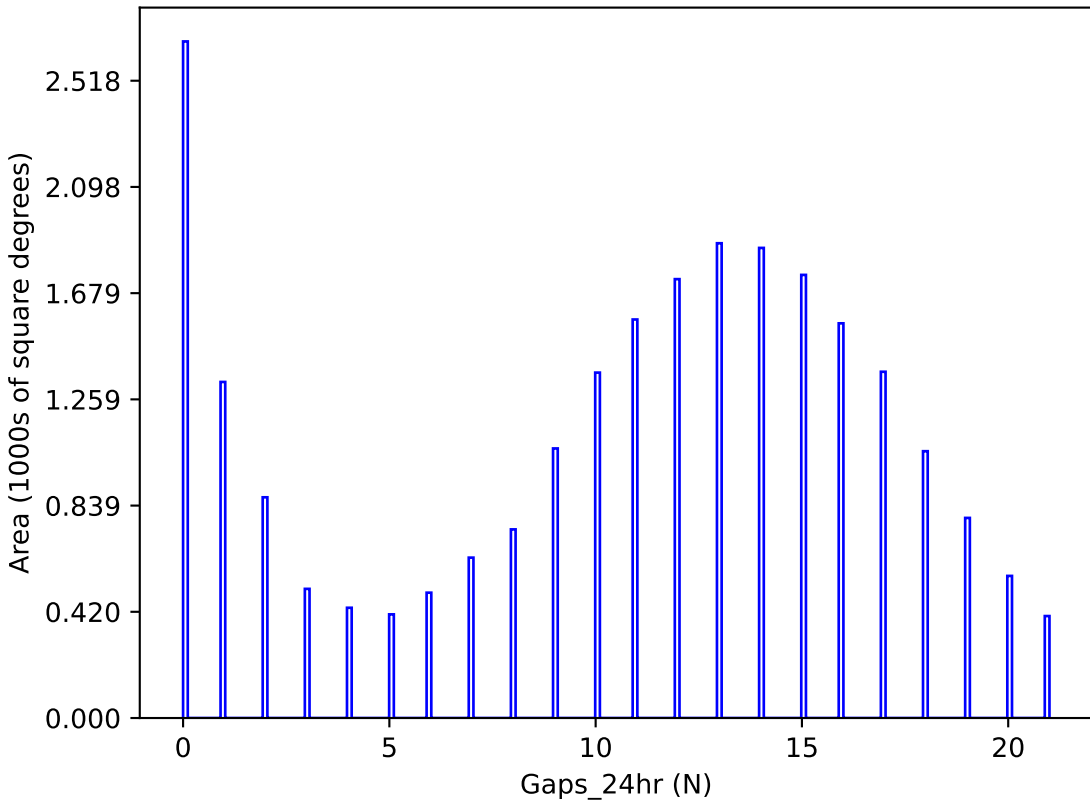
too_elab_r64_d3_ugrizy_v3.4_10yrs y band: Gaps_24hr
